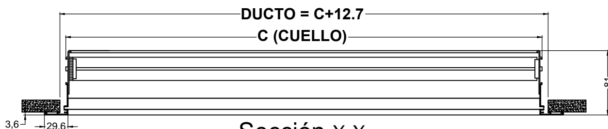
Sección X-X
