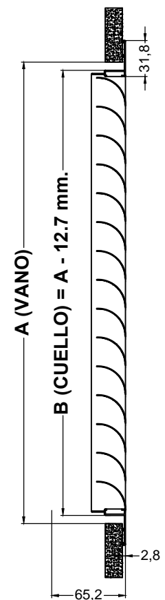
Sección x-x
